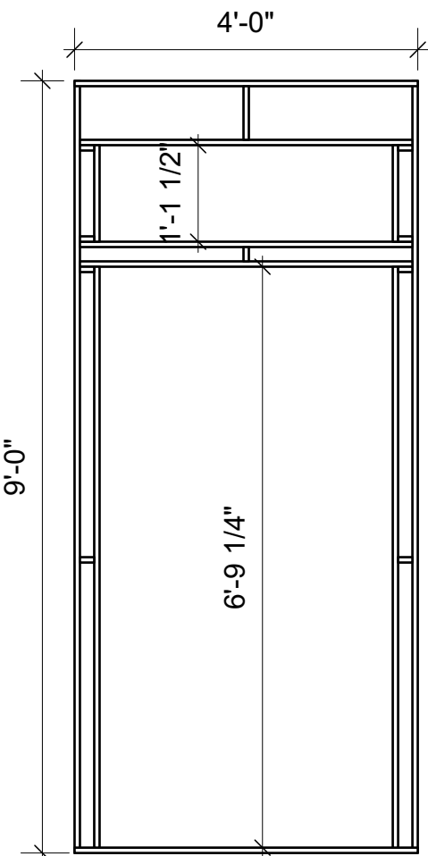
FRAME ELEVATION
