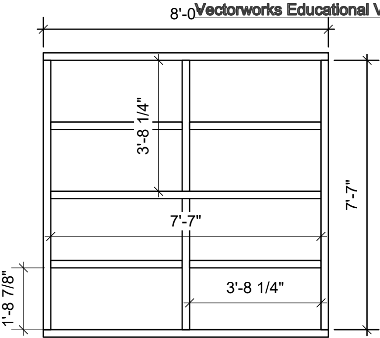
Frame Elevation
