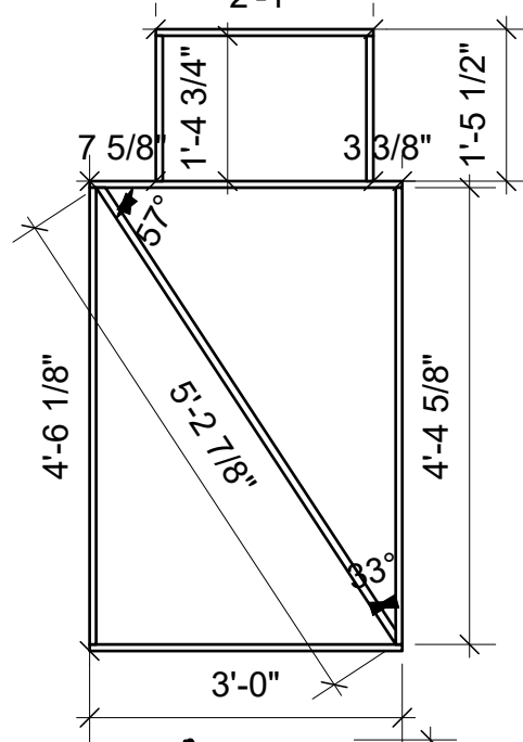
Door 2 Frame Elevation
